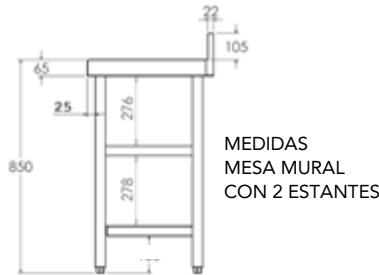
MEDIDAS MESA MURAL CON ESTANTE
