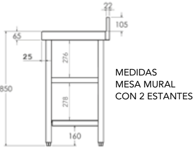
MEDIDAS MESA MURAL CON ESTANTE
