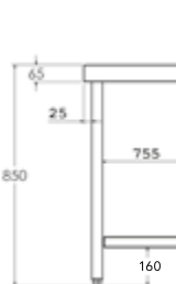
MEDIDAS MESA MURAL CON ESTANTE
