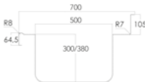
MEDIDAS CUBETA
