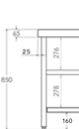
MEDIDAS MESA MURAL CON 2 ESTANTES
