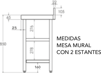
MEDIDAS MESA MURAL CON ESTANTE
