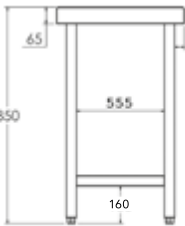
MEDIDAS MESA CENTRAL CON ESTANTE
