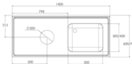
MEDIDAS FREGADERO 1400 MM
