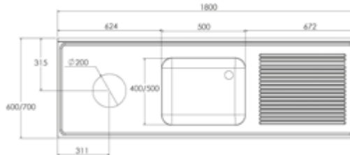
MEDIDAS FREGADERO 1800 MM
