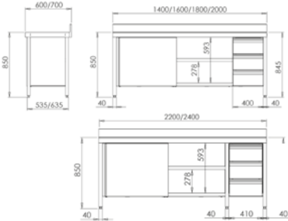
MEDIDAS MESA MURAL CON PUERTAS Y CAJONES
