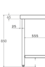
MEDIDAS MESA MURAL CON ESTANTE
