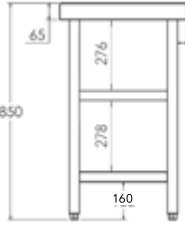
MEDIDAS MESA CENTRAL CON 2 ESTANTES
