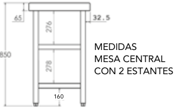
MEDIDAS MESA CENTRAL CON ESTANTE
